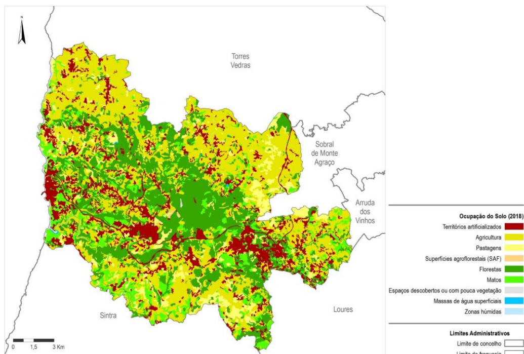
Figura 4.2. Carta de Uso e Ocupação do Solo 2018 do Município de Mafra
