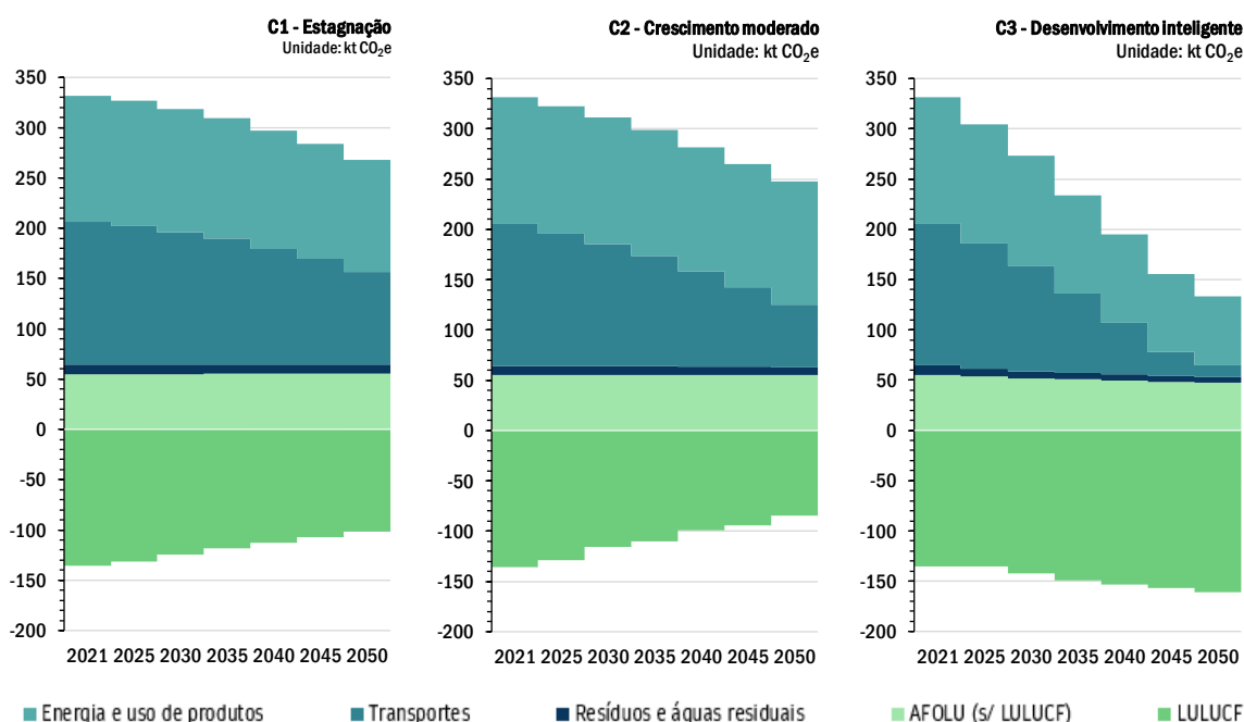
Figura 6.3.2. Contribuição por setor para as trajetórias de emissões de GEE no Município de Mafra
