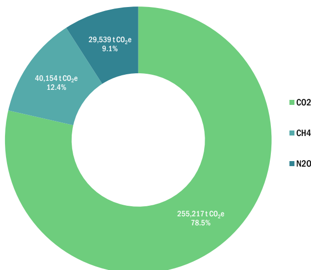
Figura 6.2.3. Emissões por tipo de GEE em Mafra (2021)
