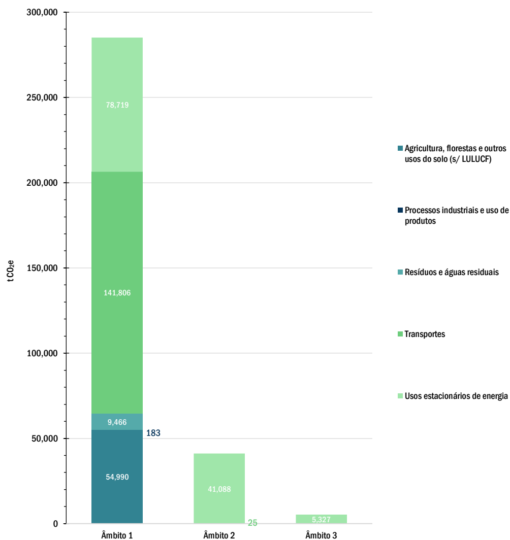
Figura 6.2.2. Emissões de GEE por âmbito e setor, sem LULUCF, em Mafra (2021)
