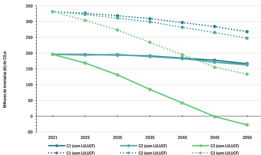
Figura 6.3.1. Trajetórias de emissões de GEE para o Município de Mafra
