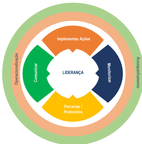
Figura 10.1. Modelo de Gestão e Acompanhamento do PMAC Mafra 2030
