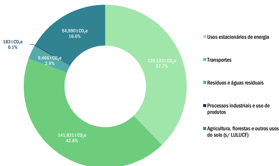
Figura 6.2.1. Emissões de GEE por setor, sem LULUCF, em Mafra (2021)
